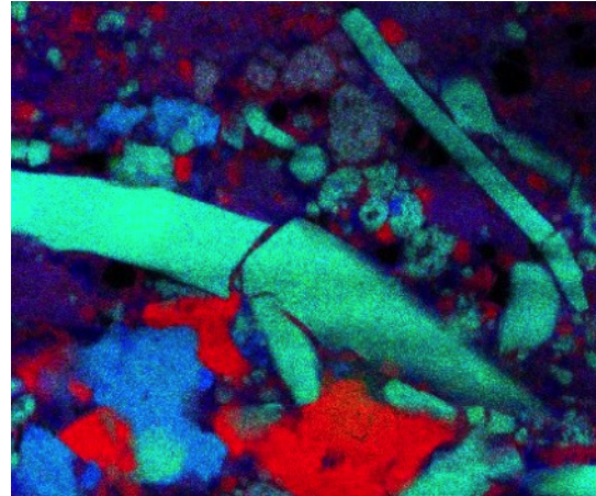
Cartographie chimique d'un assemblage de silicates et de sulfures de fer (magnésium en vert, calcium en bleu et fer en rouge).
